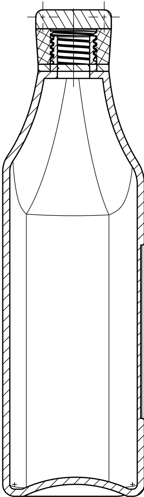
A-A (1:1)
